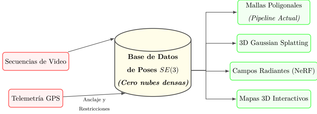
FIGURA 4.5: Arquitectura de la Base de Datos de Poses. Al almacenar y alinear el grafo espacial en lugar de puntos tridimensionales masivos, el sistema actúa como un núcleo topológico versátil que puede alimentar múltiples tecnologías de reconstrucción a futuro.
